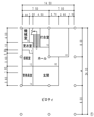
事務棟 1階 186㎡ S=1/400
