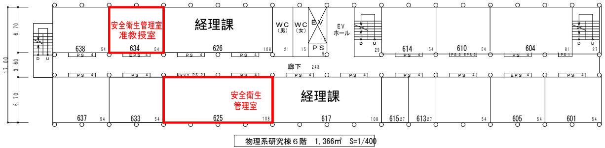
物理系研究棟 6階 1,366㎡ S=1/400
