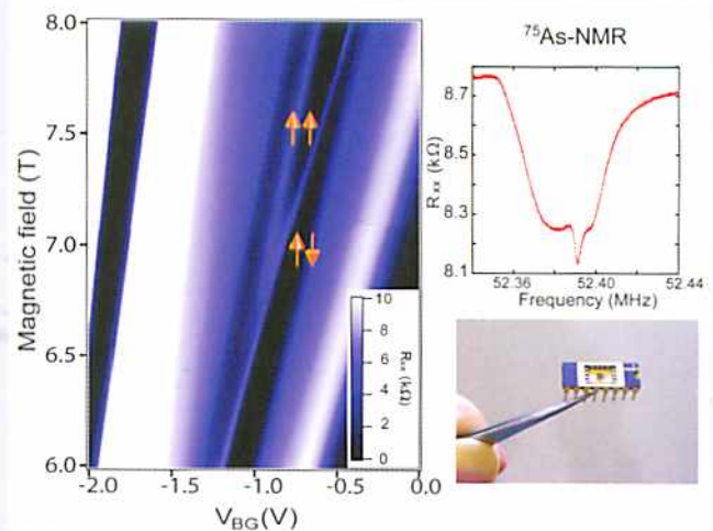
充填率2/3における分数量子ホール効果のスピン状態転移とそれを利用して測定されたNMR（核磁気共鳴）スペクトルの一例。右下は実際に測定に用いる半導体チップ。中央の小さな部分が心臓部の半導体構造である。
