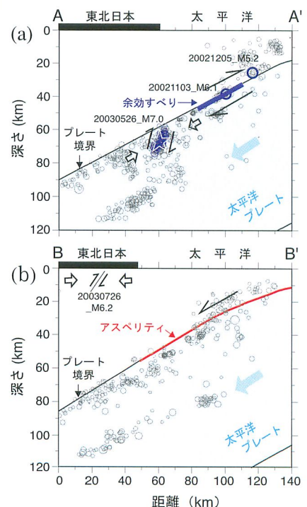
【図4】(a)図3のA-A'に沿う鉛直断面。余効すべり域を青太線で示す。5月26日の地震の震源を合わせて示す。(b)B-B'に沿う鉛直断面。宮城県沖地震のアスペリティを赤太線で示す。7月26日の地震の位置を合わせて示す。黒矢印は断層運動の向き、白矢印は圧縮力の向き。
