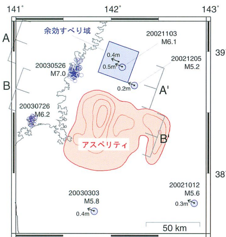
【図3】想定宮城県沖地震のアスペリティ(赤センター)周辺で発生した最近の活動。M5以上の地震と余効すべり域を示す。矢印はプレート境界のすべりを示す。5月26日および7月26日の地震を合わせて示す。
