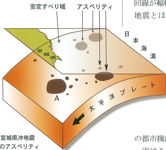
【図1】プレート境界におけるすべり様式の模式図。アスペリティ(固着域)は通常は固着している、地震時に急激にすべる。安定すべり域は、地震と次の地震の間あるいは地震後にゆっくりとすべり、地震時にはむしろ急激なすべりを抑制する動きをする。
