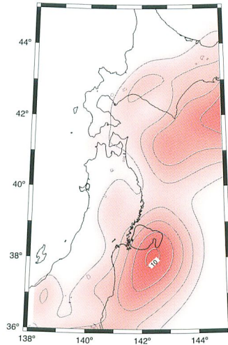
【図2】GPSデータを用いて推定されたプレート境界の固着状況[諏訪・他,2003]。プレート間の固着の度合いを表すバックスリップ量をコンターで示す。コンター間隔は2cm/yr。宮城県沖地震のアスペリティを黒太線で示す。
