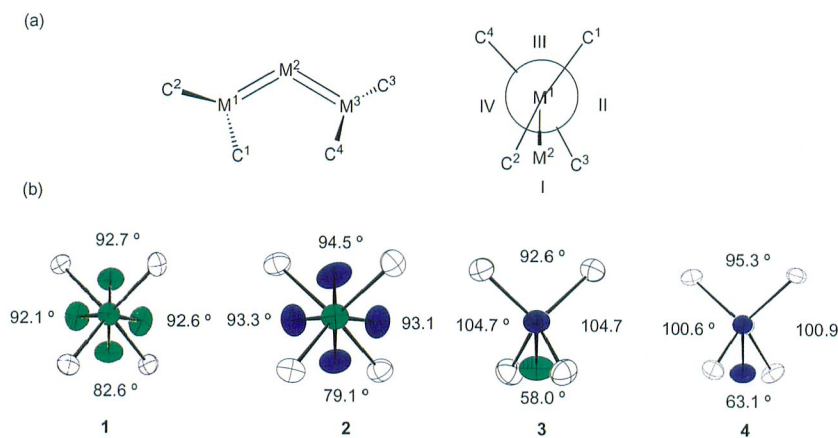
図2. (a) 高周期14族元素アレンの4つの象限I-IVの模式図 (b) 高周期14族元素アレン1-4の両端原子が重なるようにして見たアレン骨格の図
