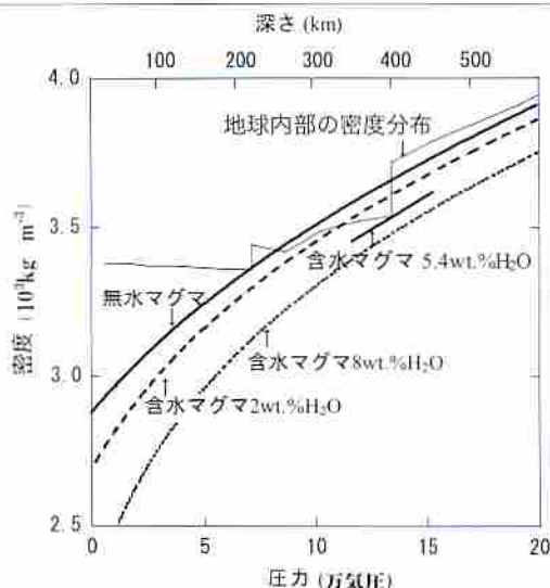
図4 含水マグマと標準マントル(PREM)との密度の比較。5.4wt.%までH 2 Oを含むマグマは周りのマントルよりも重く安定に存在する。
