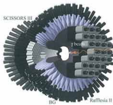
大立体角ガンマ線検出器: FOREST
