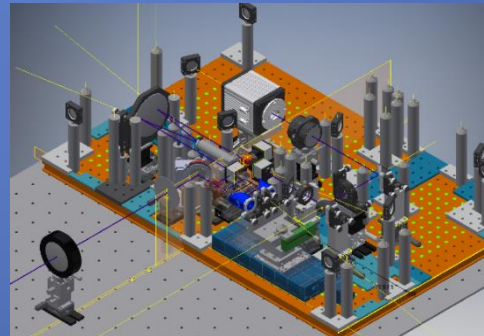
すばる望遠鏡用波面センサーのモデル図(左上) と実際に組み上げている様子(右上 photo:志鎌康平)
