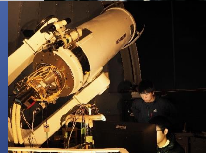
すばる望遠鏡用波面センサーのモデル図(左上) と実際に組み上げている様子(右上 photo:志鎌康平)
