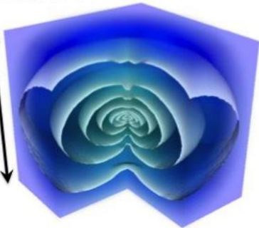
(a) 原始星形成時
