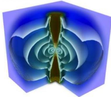
(b) 25太陽質量 (2万年後)
