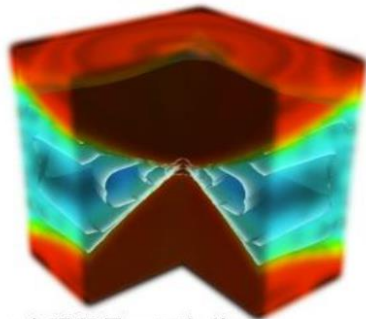
(d) 42太陽質量 (7万年後)
