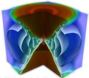
(c) 32太陽質量 (3万年後)
